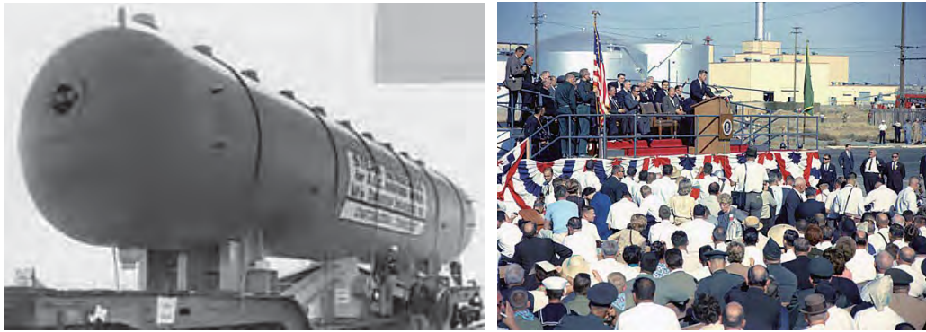
図 11. N 原子炉の蒸気生成機と蒸気生成機を捧げるケネディ大統領
