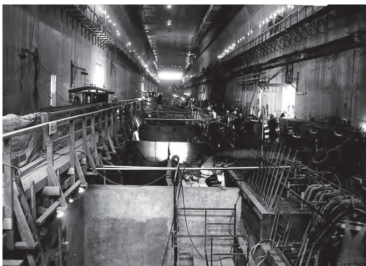
図3. PUREX 使用済み核燃料再処理工場
